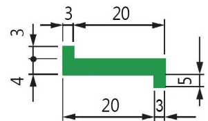
■ GP 262 大Z Profile 45M/Roll 型墊片 45M/捲
